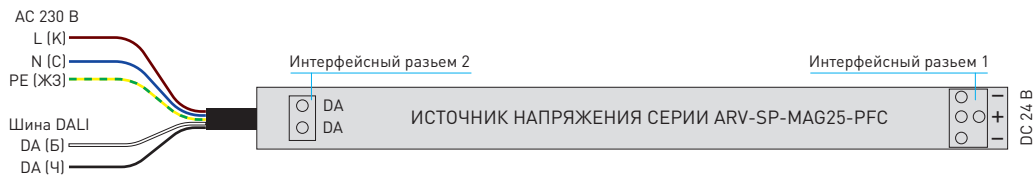
Рис. 1. Схема подключения
